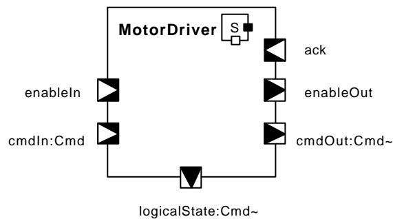
Figure 9 « s_capsule » du MotorDriver
